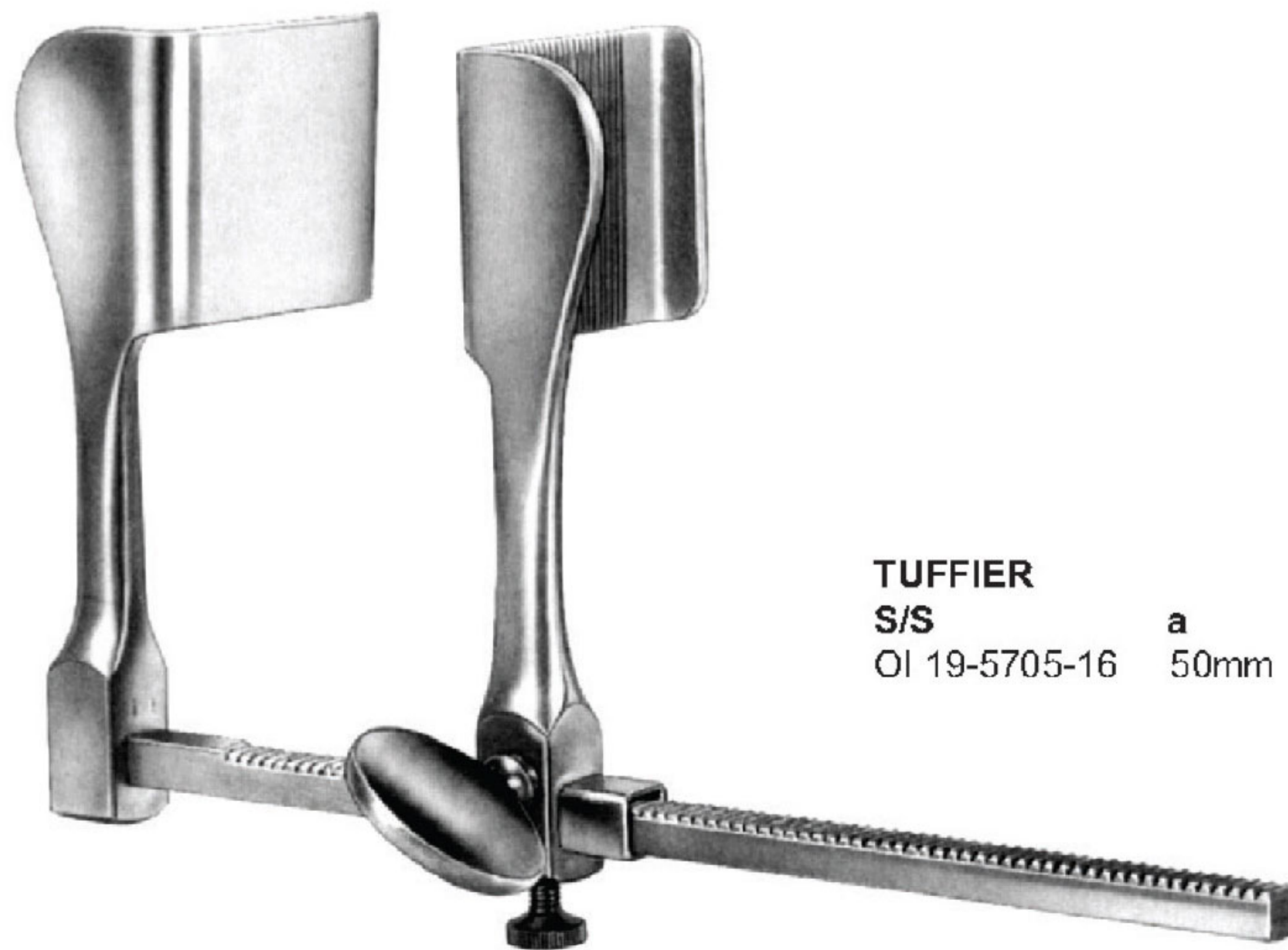
TUFFIER S/S Ol 19-5704-17 a 43mm b 53mm c 130mm
